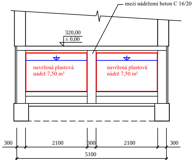
ŘEZ C - C'
